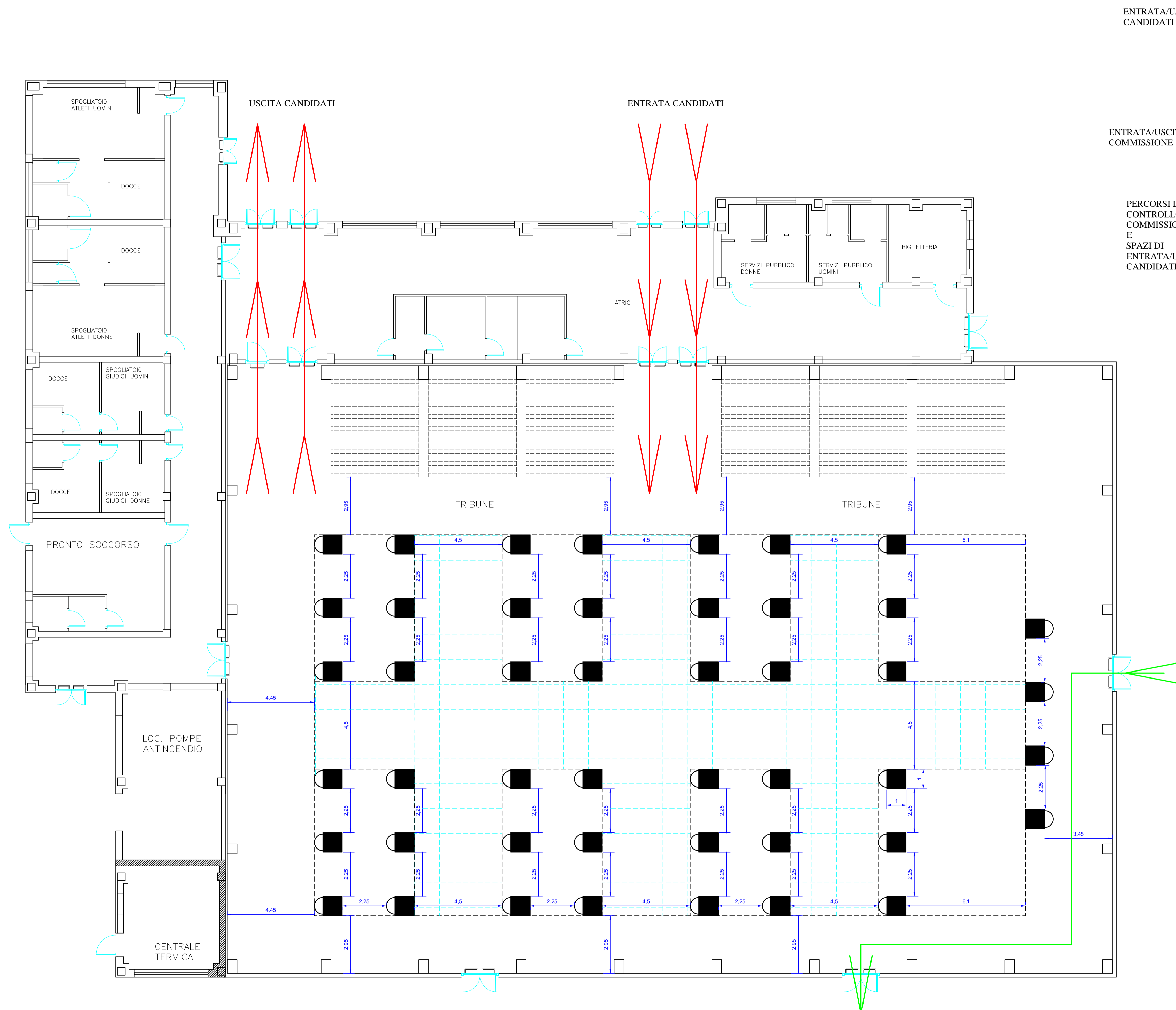
PLANIMETRIA sc. 1:100
